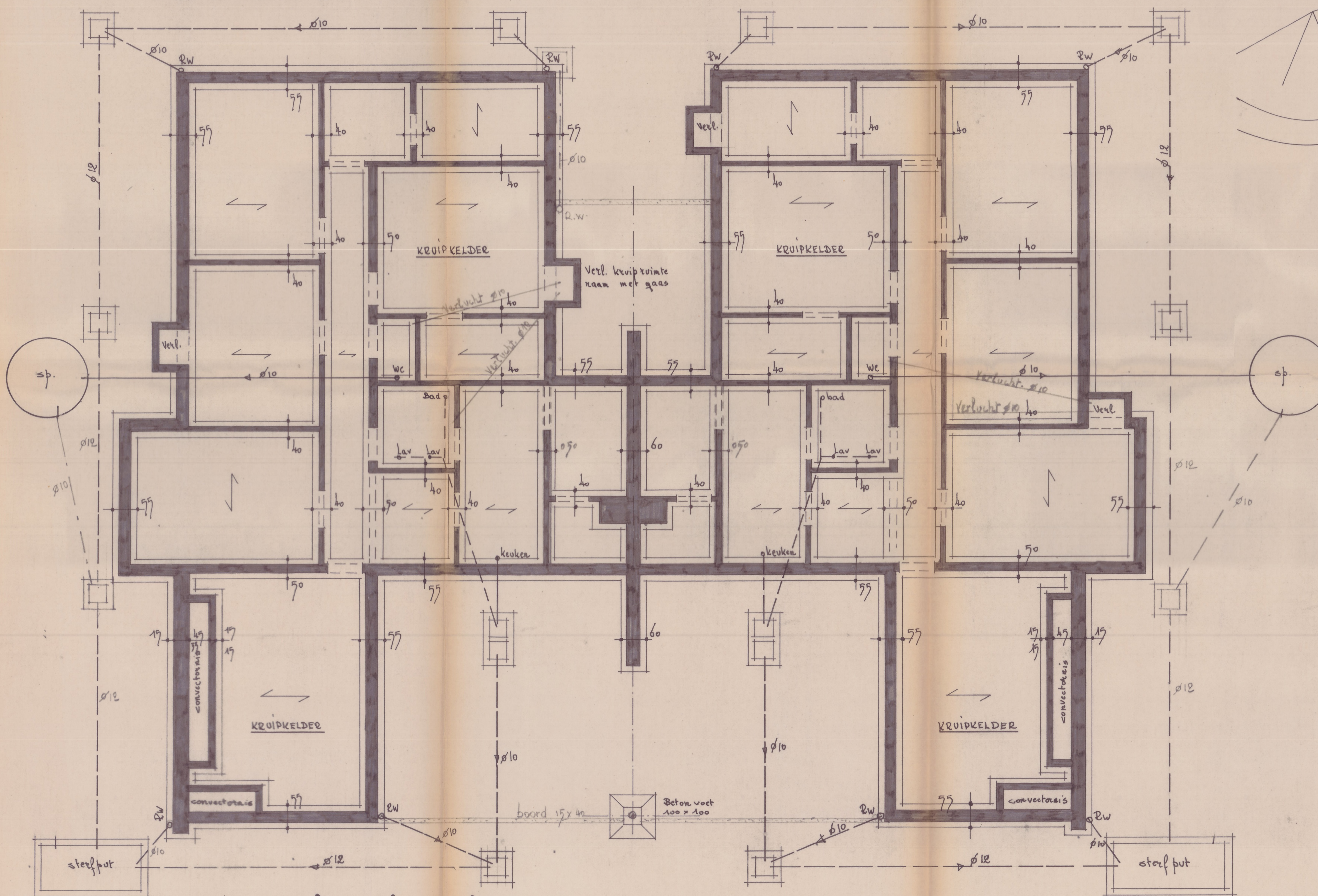
FONDATIE-RIOLERING.
